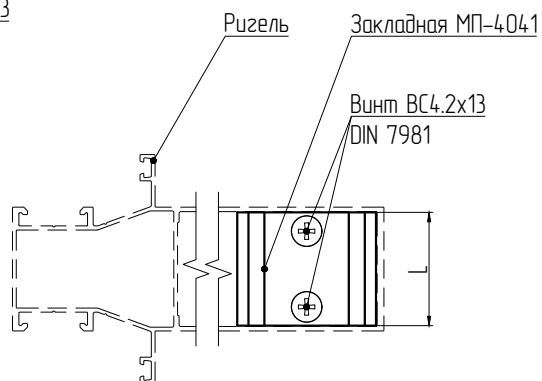
Выбор длины закладной МП-4041 для усиленного Т-образного соединения
