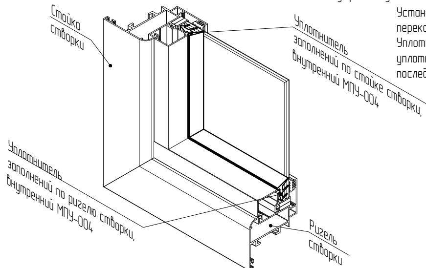
Шаг 5. Установка внутренних уплотнителей
